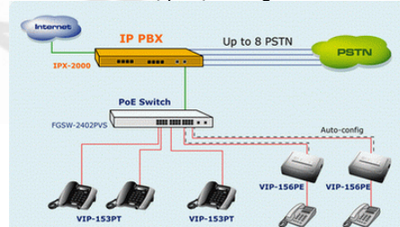
Giải pháp mô hình truyền thông ngang hàng VIP-156PE (Home / SOHO)
