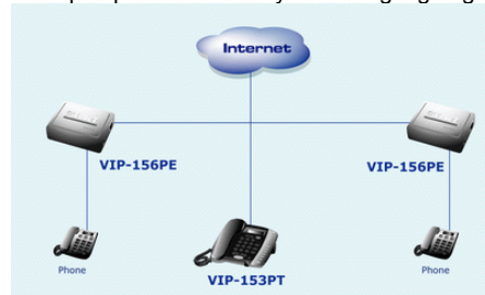
Giải pháp mô hình truyền thông VIP-156PE qua SIP proxy (giải pháp của nhà cung cấp dịch vụ)
