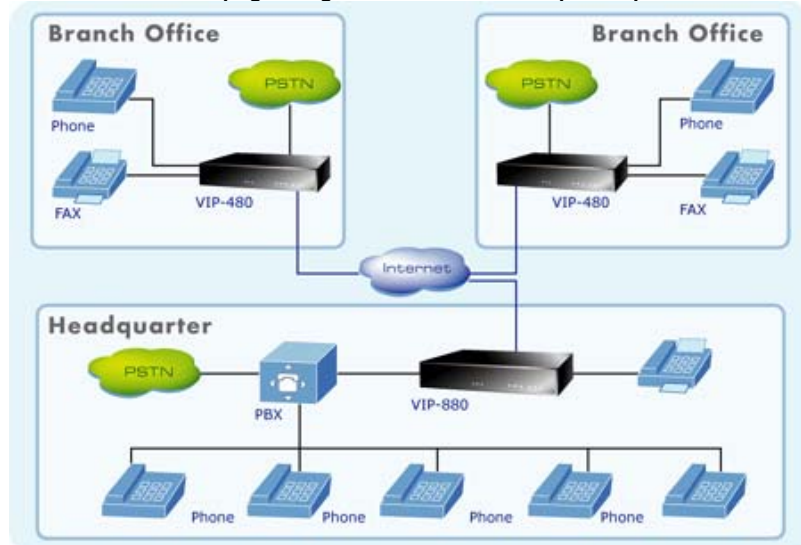
VIP-880FO sử dụng trong mô hình kết nối điện thoại IP đa điểm
