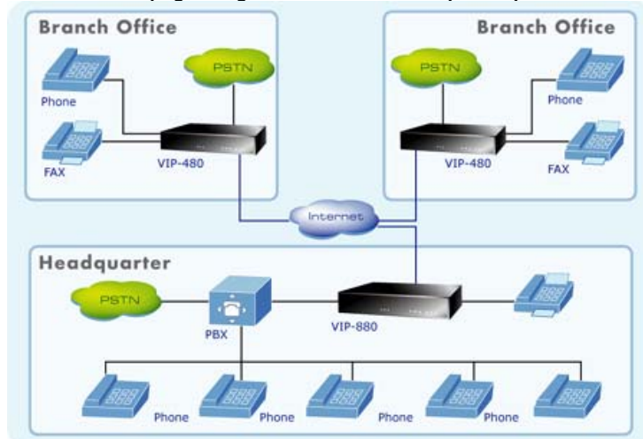
VIP-880 sử dụng trong mô hình kết nối điện thoại IP đa điểm
